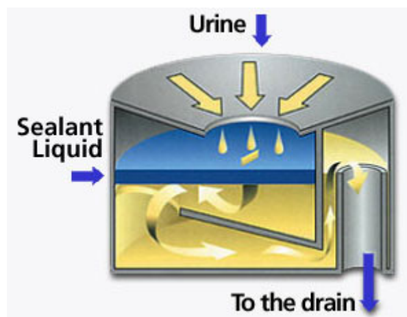
Obr. 1 Kartridž s biodegradabilní tekutinou (modrá) zabraňující pronikání zápachu moči (žlutá) do okolí. (Zdroj: firemní stránky Falcon Waterfree Technologies).
